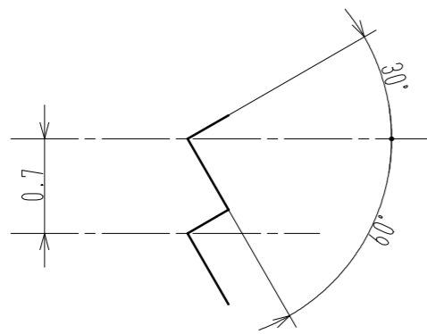
ヤスリ目断面(File surface) scale 20:1
